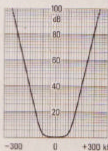
Selectivitetskurve for FM-mottakeren.
