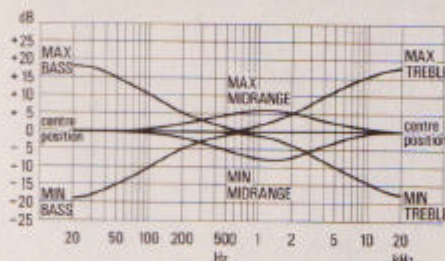
Frekvenskurver med bass-, mellomtone- og diskant-kontr. i minimum-, midt- og maksimumsstillinger (uten frekvenskorrigering).
