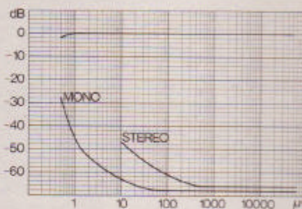
Signal-støy forhold i stereo og mono for FM-mottakeren.
