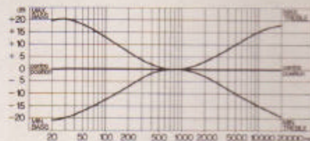
Frekvenskurver med bass- og diskantkontroller i maksimum-, midt- og minimumsstillinger (uten frekvenskompensering).
